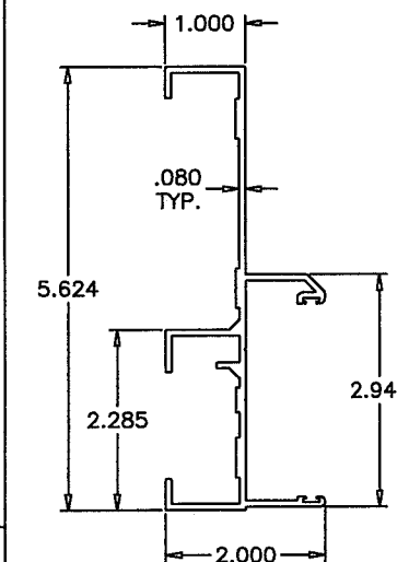
③ FRAME JAMB
